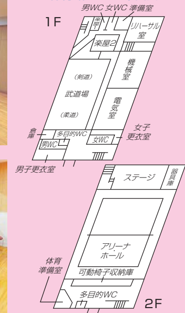
体育館・ホール平面図
